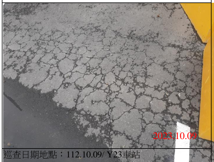
巡查日期地點：112.10.09/ Y23車站 照片說明：路面龜裂狀況
